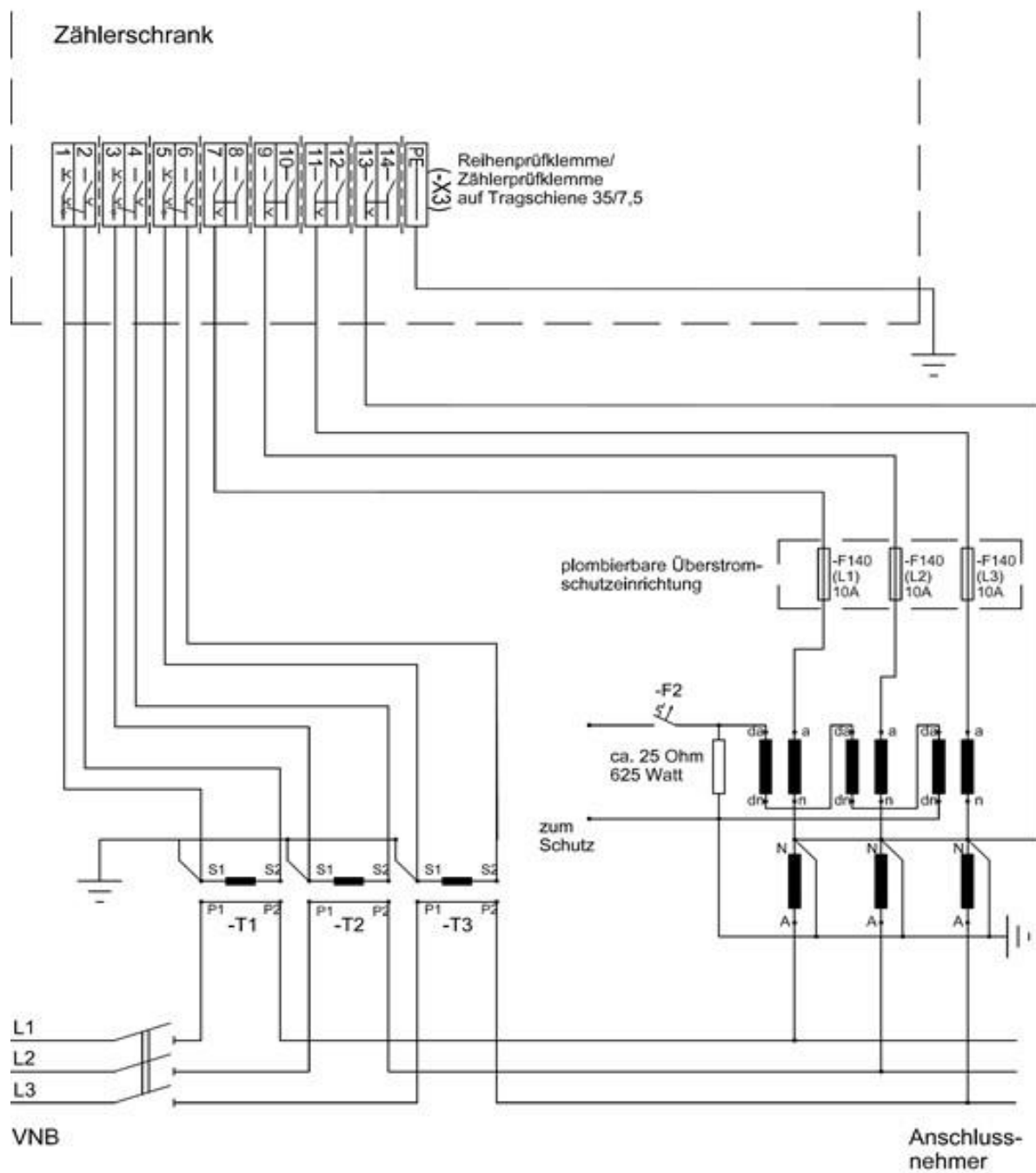
Abb. 40: Messschaltung für die mittelspannungsseitige Abrechnungszählung
