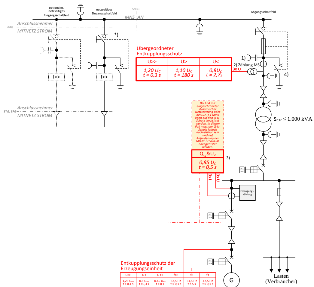
Abb. 30: (ehemals D5a): \leq 20 -kV-Anbindung einer Mischanlage über einen Transformator
