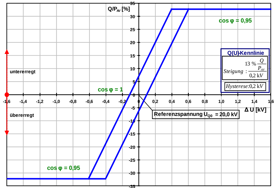
Abb. 49: Q(U) -Kennlinien-Regelung (ehemals Bild L.1)
