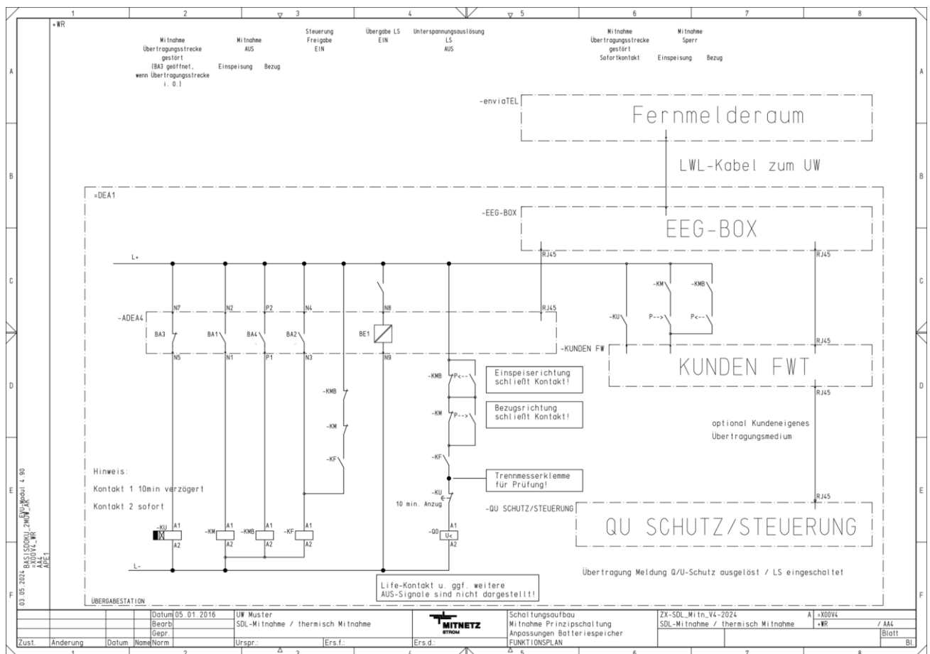
Abb. 48: Schaltungsaufbau der LWL-Kabelverbindung zwischen der Übergabestation und dem NG Forst Lausitz-Umspannwerk (richtungsabhängig)
