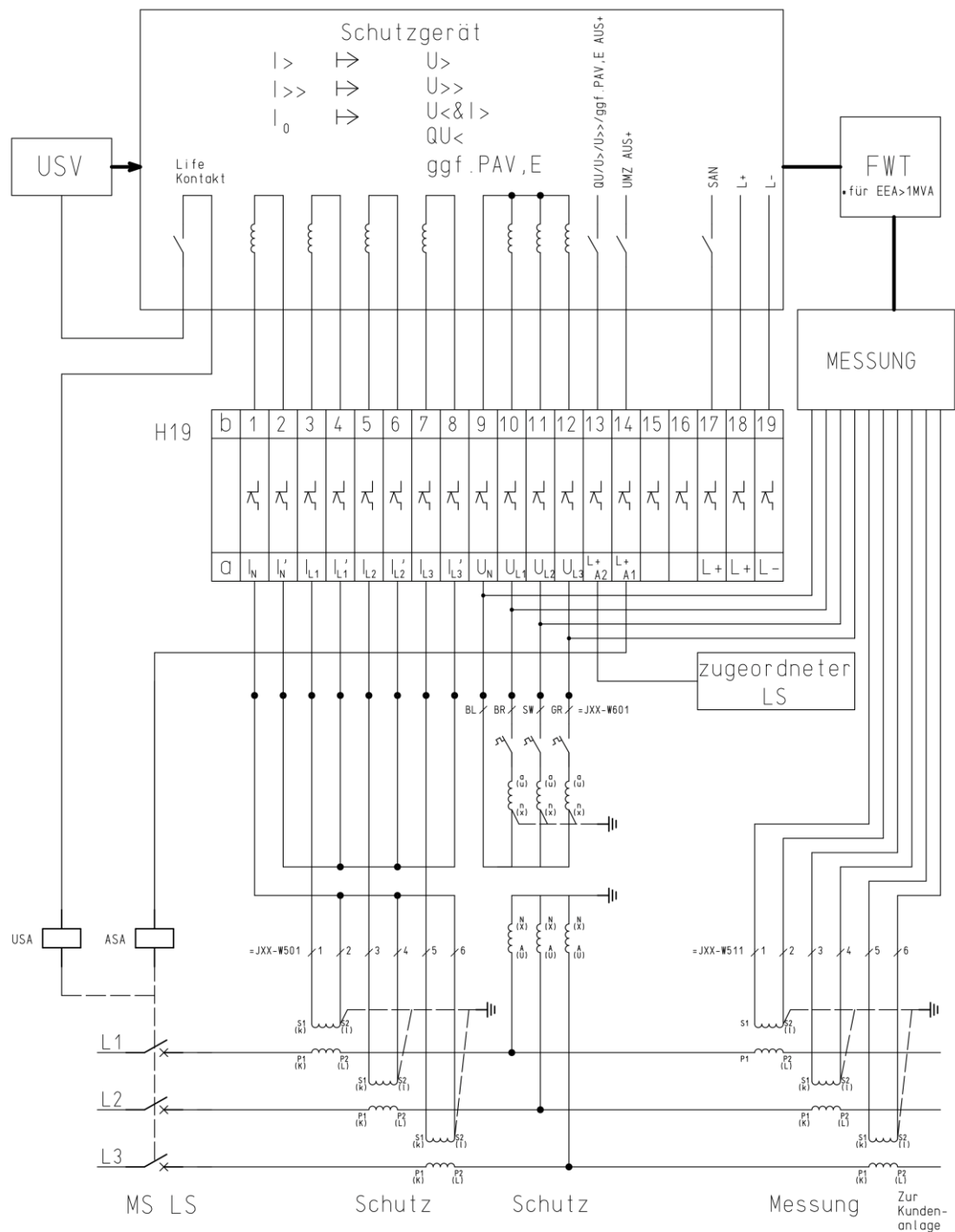
Abb. 42: Wandlerverdrahtung Anbindung UMZ / übergeordneter Entkopplungsschutz
