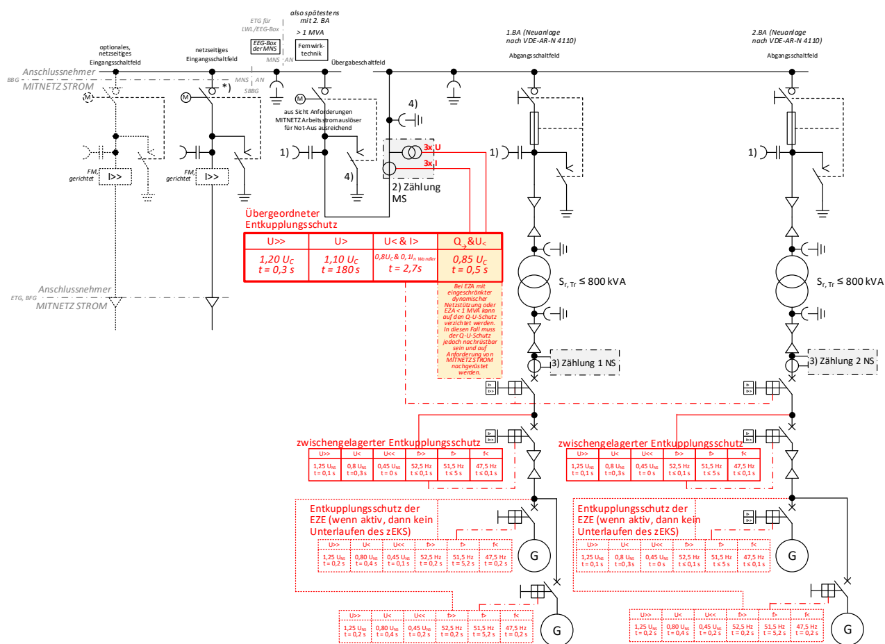
Abb. 29: (ehemals D4e): ≤ 20-kV-Anbindung von zwei Bauabschnitten einer PV-Anlage mit je 750 kVA (spätestens ab 2.BA mit FWT, in diesem Fall im 1.BA mit FRE)
