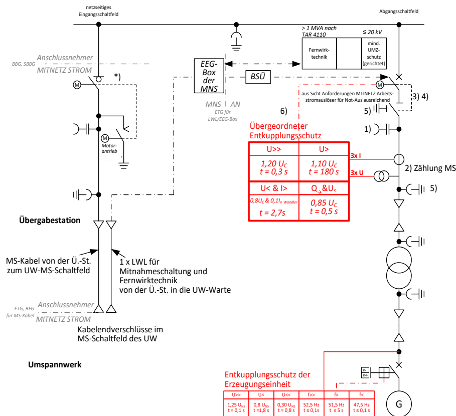
Abb. 24: (ehemals D3a): ≤ 20-kV UW-MS-Sammelschienenanschluss einer Erzeugungsanlage
