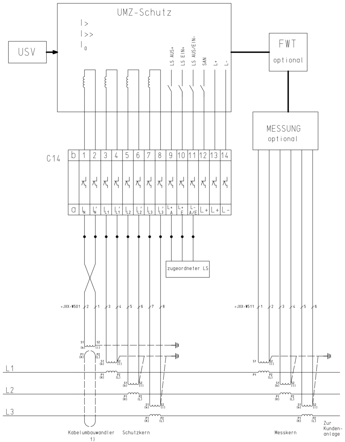
Abb. 43: Wandlerverdrahtung Anbindung UMZ-Schutz
